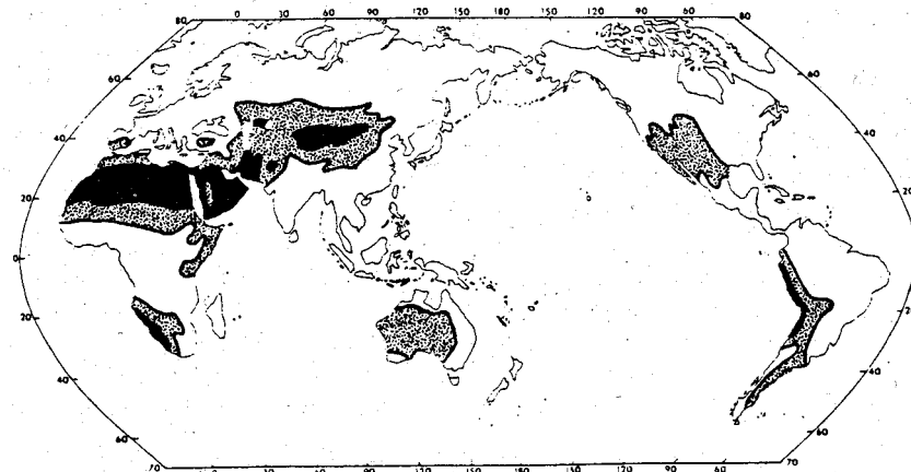
Abb.2: Weltweite Verteilung von Trockenheit Wert von 2-10 Wert von >10 (Budyko-Lettau Trockenheitsverteilungsschlüssel)
